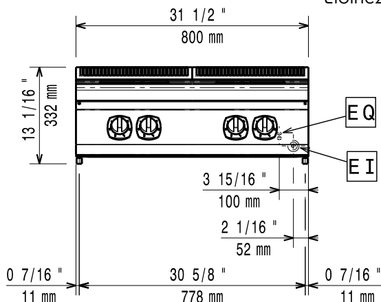
Előlnézet
